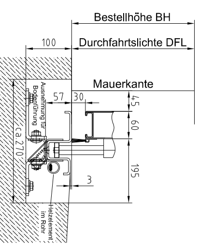
d) Bodenführung beheizt BF-light NIRO bhz.
