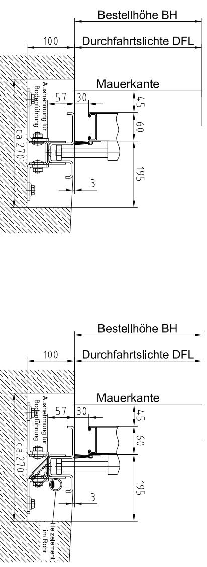
c) Bodenführung BF-light NIRO
