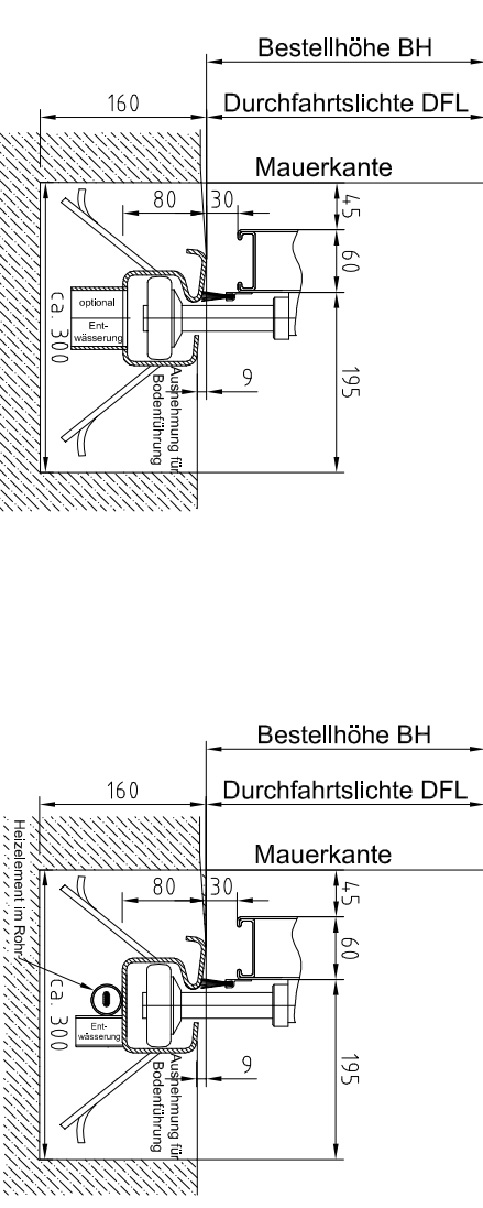
c) Bodenführung BF-light NIRO
