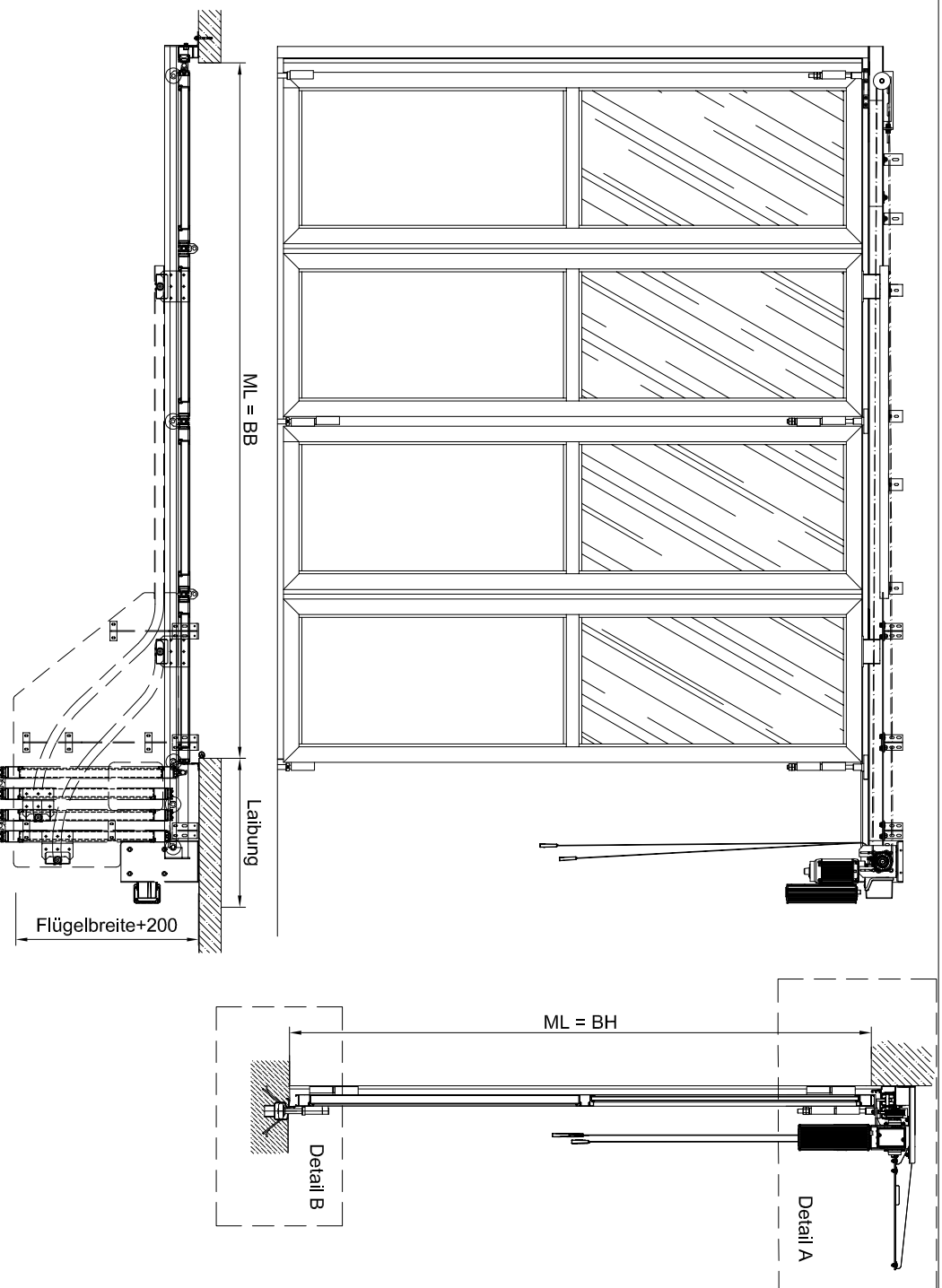
Montagesituationen im Sturz (M1:8) - Detail A ca. 950 (von Flügelbreite abhängig)
