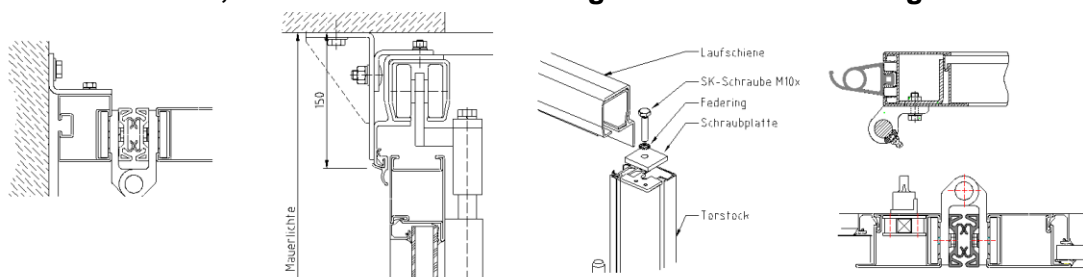
Befestigung am Mauerwerk
