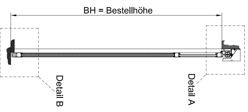
Vertikalschnitt
